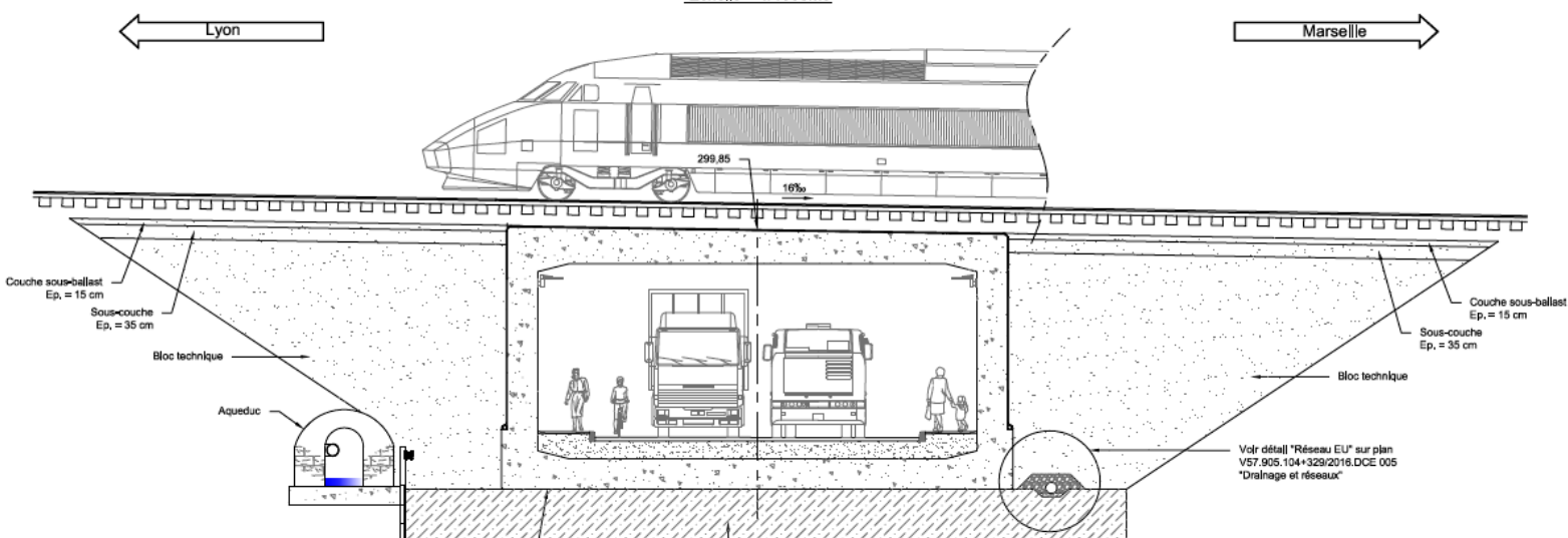
Coupe transversale de l'ouvrage projeté
