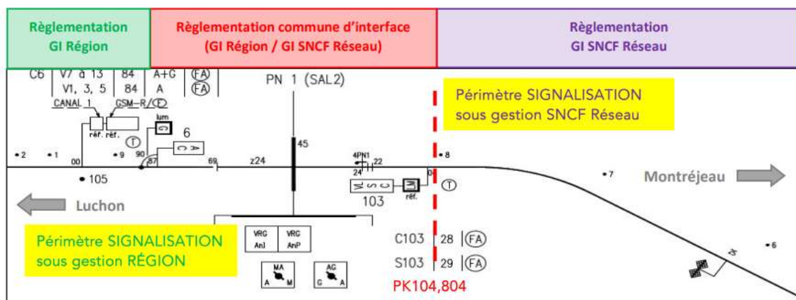
Figure 2 : Schéma du point frontière entre le périmètre Région et le périmètre SNCF Réseau de la ligne Montréjeau-Luchon
